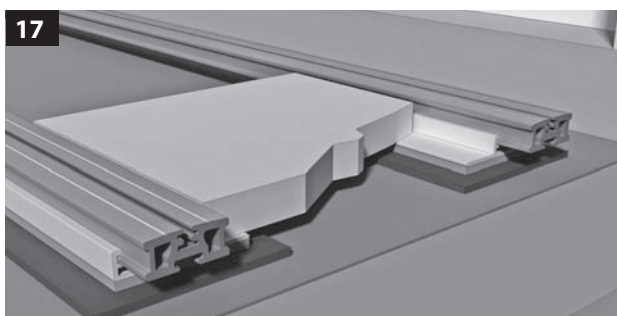
17 Plattenanker aufchieben und entsprechend der Lage und Position der Betonplatten ausrichten.
