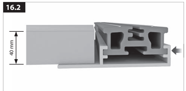
16.2 Positionierung des UK-Profils im Plattenanker (vgl. 8.2).
