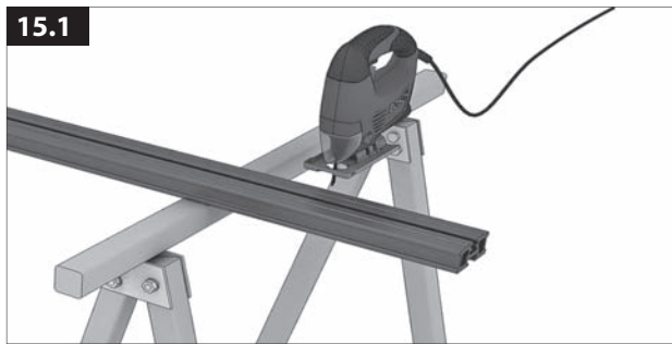
15.1 Zuschneiden der UK-Profile.
