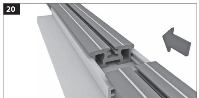
20 Verlegung der UK-Profile auf Stoß. Plattenanker im Stoßbereich unterlegen.
