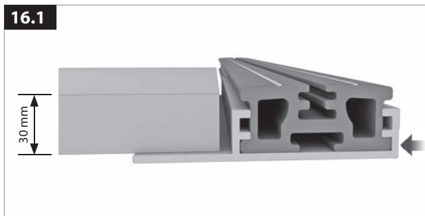
16.1 Positionierung des UK-Profils im Plattenanker (vgl. 8.1).
